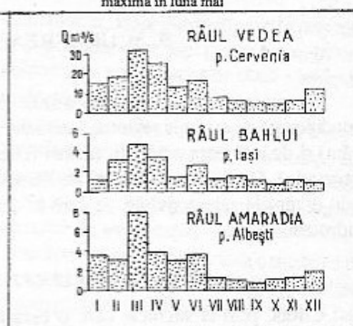
Fig. 144. Tipul de râuri Moldavo-Valah cu scurgerea maximă în luna martie.
