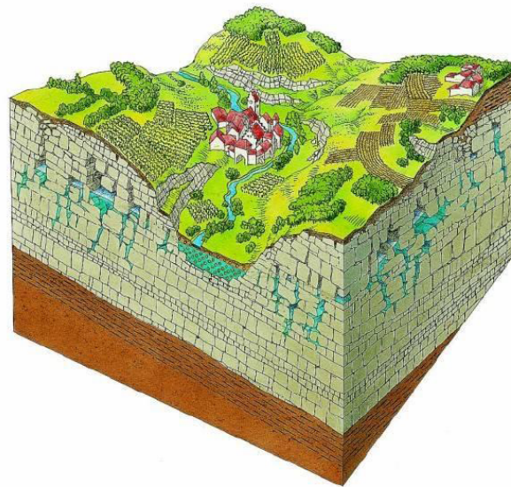
groundwater in Karst formations (Karst- grundwasserleiter)
