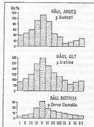
Fig. 146. Tipul de râuri carpatic cu scurgerea maximă în luna mai
