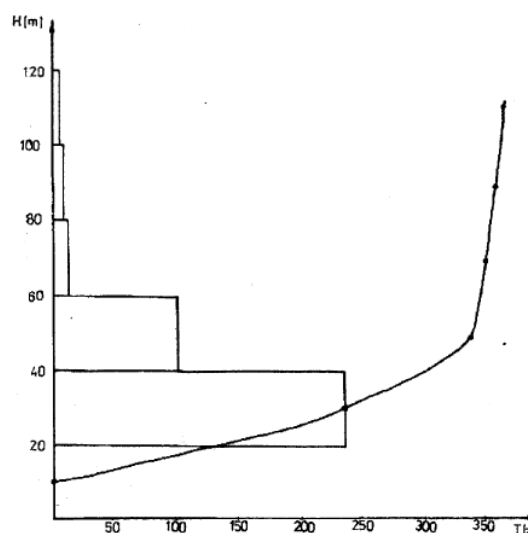
2.3 Graficul de frecvență și de durată a nivelurilor măsurate pe râul Olt, la postul hidrometric Râmnicu-V.
