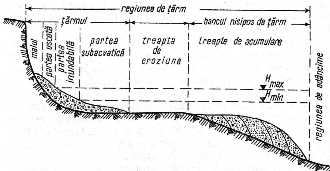
Profil morfologimnologic în regiunea de țărm.
