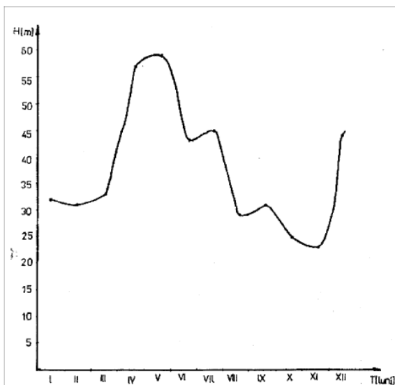
Fig. 2.2 Hidrograful nivelurilor medii lunare măsurate pe râul Olt, la postul hidrometric Râmnicu-Vâlcea
