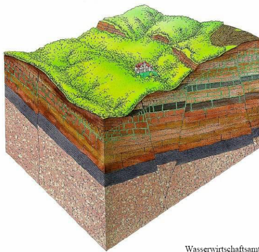
groundwater in fissured rocks (Kluftgrundwasser- leiter)
