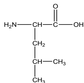
leucina
