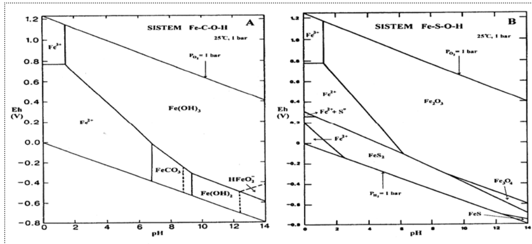
Diagrame Pourbaix la t, p normale pentru sist. (A) Fe-C-O-H, (B) Fe-S-O-H, (după Brookins, 1998)
