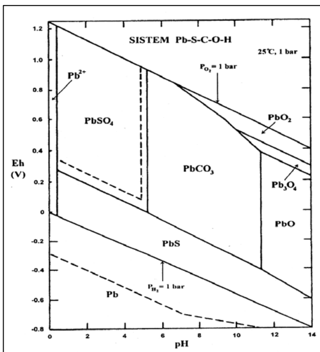
Diagrama Pourbaix pentru sistemul Pb-S-C-O-H, c.n.(după Brookins, 1998).
