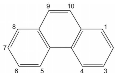
fenantren
