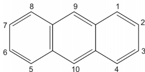
antracen
