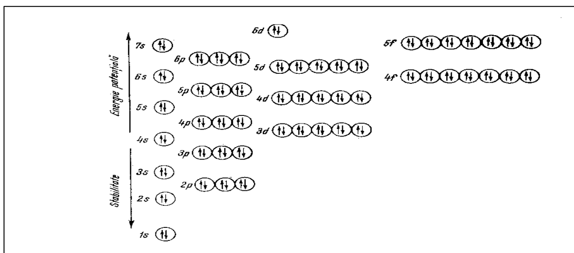
Succesiunea straturilor cu substraturile și orbitalii lor atomici (după Rabega C., 1975).
