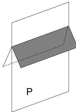
Fig. 6: Dom
