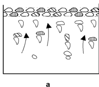
Fig. 23 - a) Migrarea ascensională a componentelor volatili spre partea superioară a camerei magmatice.
