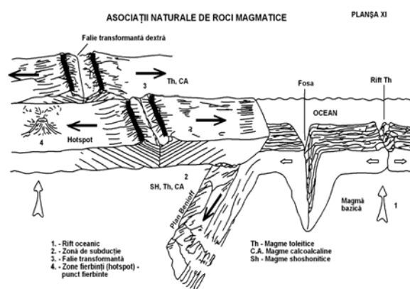
Fig. 36. - Imagine de ansamblu privind tectonica globală în plăci (după M. Bleahu, 1984 modificată de V. Popescu, 1993)
