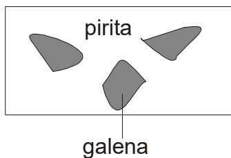
Fig. 37 - Concreștere epitaxială
