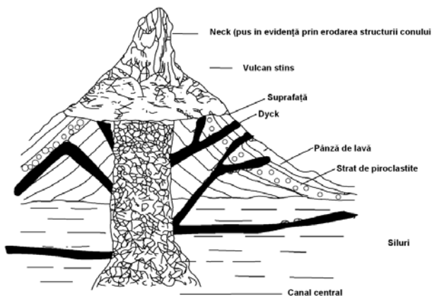
Fig. 5 - Rocile intrusiv din apropierea suprafeței care se prezintă sub formă de structuri magmatice - după Sokolov, 1967, modificată de V. Popescu, 1993
