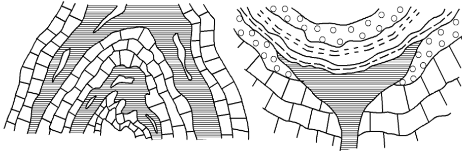
Fig. 10 - Facolite
