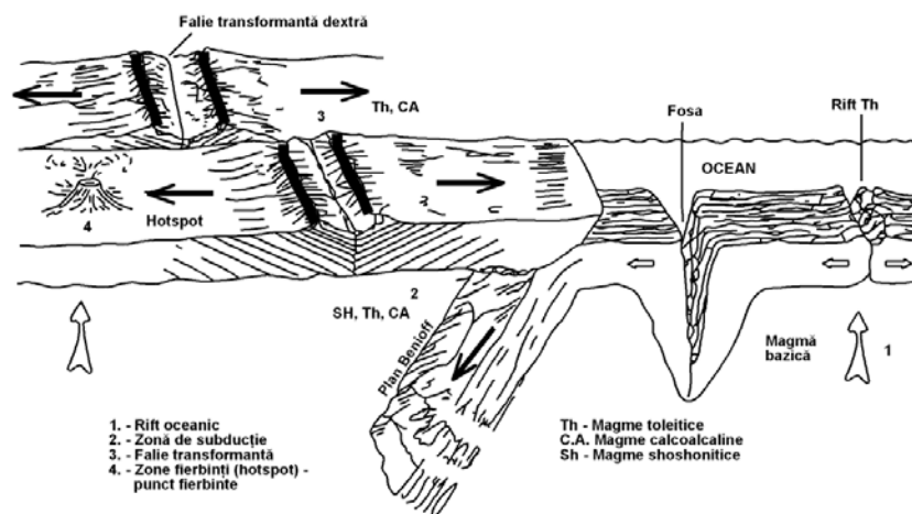
Fig. 36. - Imagine de ansamblu privind tectonica globală în plăci (după M. Bleahu, 1984 modificată de V. Popescu, 1993)
