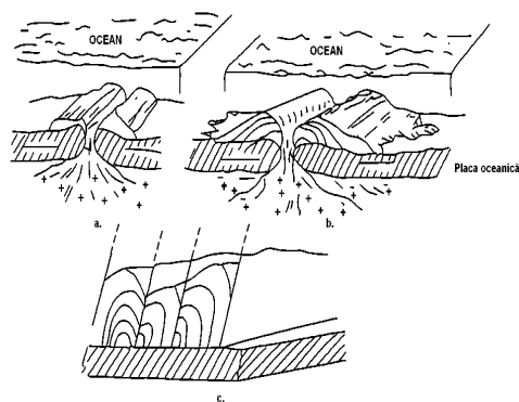
Fig. 38 - Momente ale coeziunii și închiderii bazinelor oceanice:
