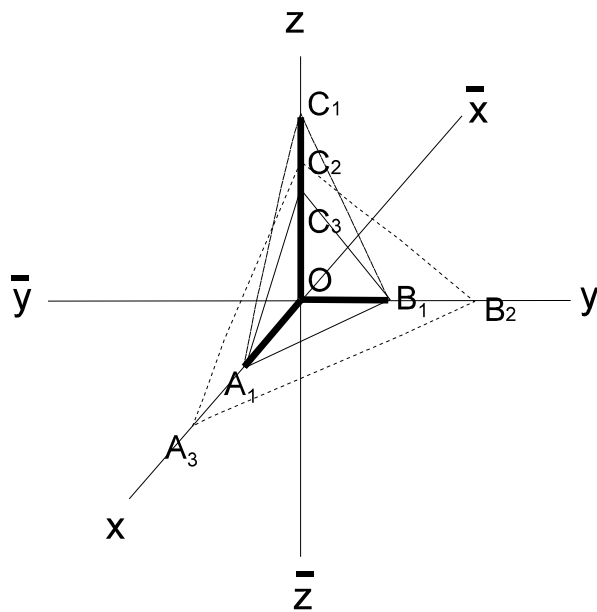
Fig. 17 - Definirea poziției unei fețe
