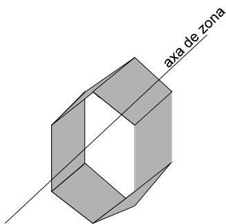
Fig. 21 - Axa zonei
