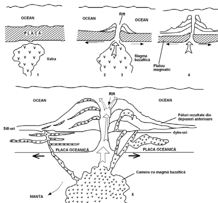
Fig. 28 - Generarea magmelor bazaltice în zona de rift (1, 2, 3, 4, 5)
