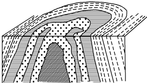
Fig. 12 - Dyke inelar
