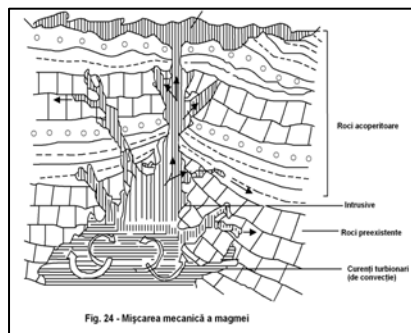
Fig. 24 - Mișcarea mecanică a magmei
