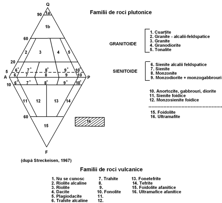
Fig. 32 Clasificarea generală și nomenclatura rocilor plutonice și vulcanice (după recomandarea I.U.G.S., 1967)
