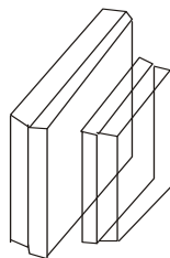
Fig. 35 - Macla albit - Karlsbad - ortoză
