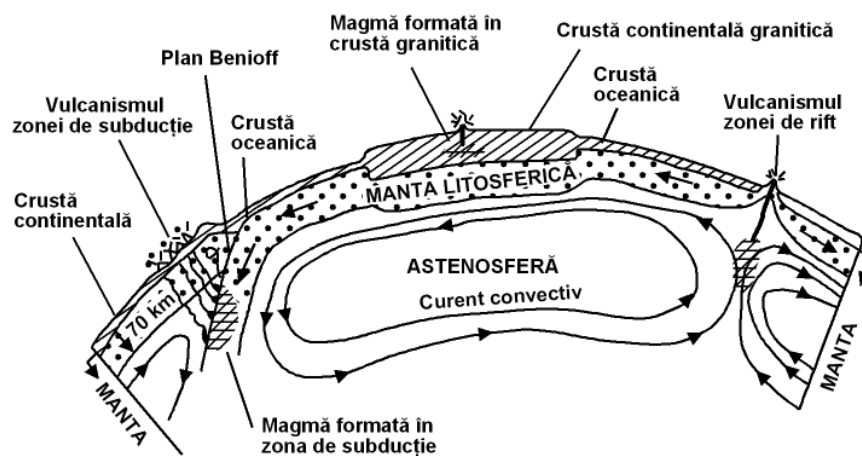
Fig. B - Condițiile geologice cele mai favorabile generării magmelor prin anatexie - după N. Anastasiu, M. Șeclăman - 1984
