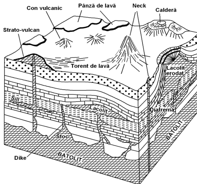
Fig. A - Principalele forme de zăcământ ale rocilor magmatice (după Șeclăman et al., 1999)
