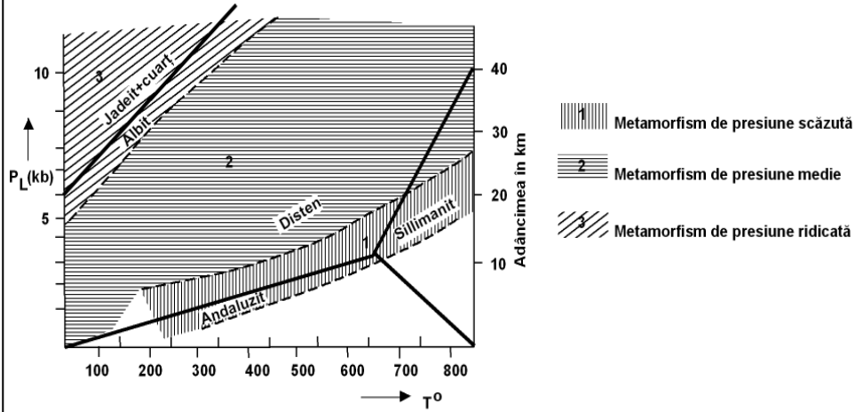
Fig. 65 - Dispunerea mineralelor într-o parageneză metamorfică
