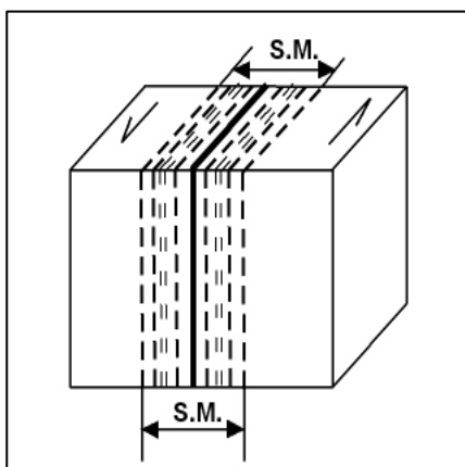
Fig. 1 - Poziția S.M. în zona de forfecare (săgețile indică direcția și sensul deplasării relative a unităților vecine (după Șeclăman et al., 1999)
