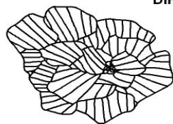
Fig. 63 - Concreționarea metamorfică (porfiroblast)
