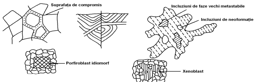
Fig. 61. - Tipuri de cristale: poliedrice, xenomorfe, porfiroblaste idiomorfe sau xenoblaste
