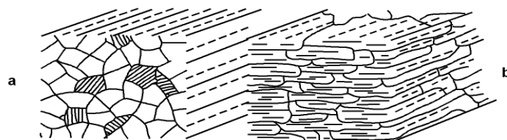
Fig. 62 - Formarea șistuoziității de tip: a. - linear; b. - planar
