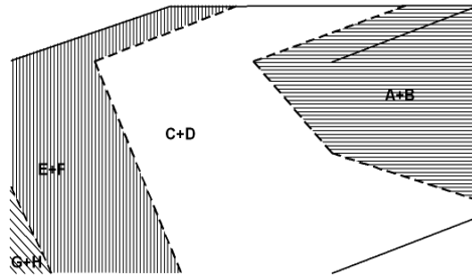
Fig. 67 - Zone de metamorfism
