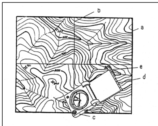
Fig. 147. Transpunerea pozițiilor pe hartă cu busola (metoda azimutului căderii): a – cadrul lateral (N – S) al hărții; b – caroiajul geodezic; c – busola; d – latura sudică a plăcii rabatabile; e – poziția marcată graphic (după Basarab și al., 1995)
