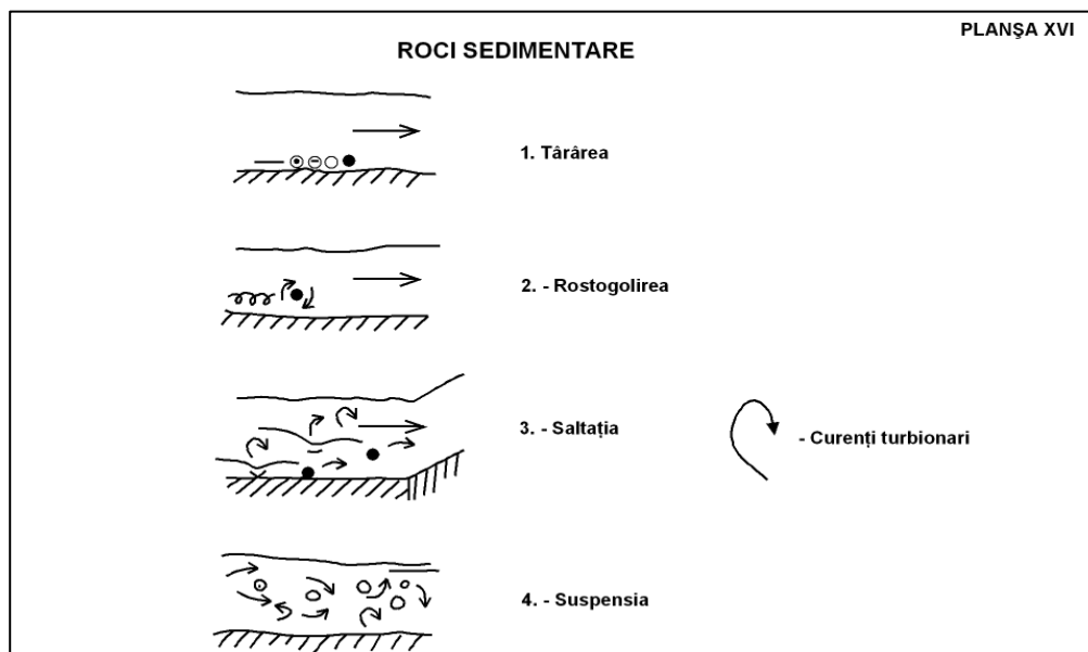
Fig. 47 - Deplasarea sedimentelor de fund (după Otiman, 1965 și Dimitriu, 1967)
