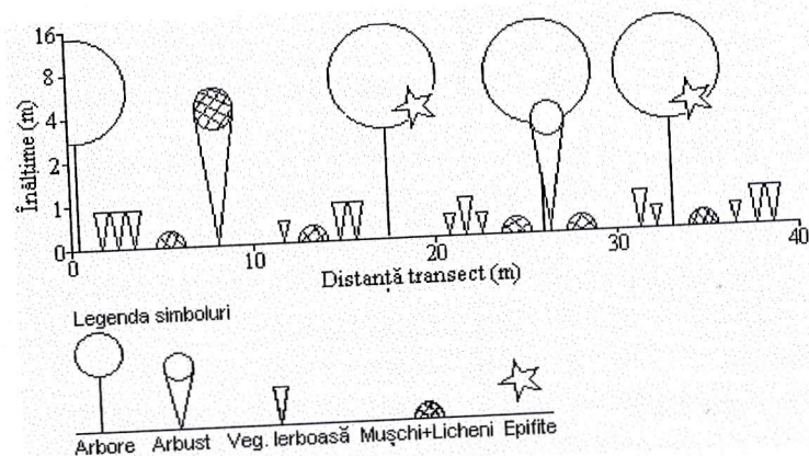
Figura.15. Profil de vegetație de-a lungul unui transect liniar (Williams,1994).
