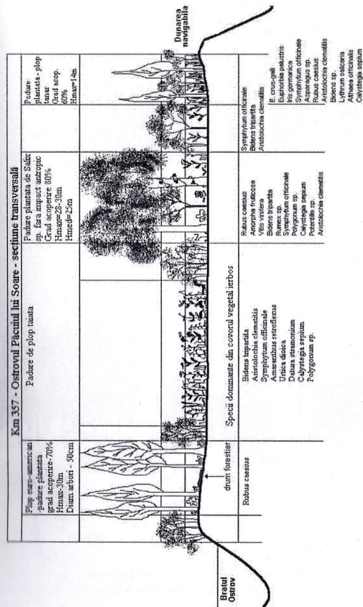
Figura 16. Profilul vegetației (fără scară) de-a lungul unui transect liniar în ostrovul Păcuilui Lui Soare, pentru evidențierea succesiunii spațiale a diferitelor tipuri de comunități vegetale (Topa Sorana, Cheorghie Iuliana, date nepublicate).
