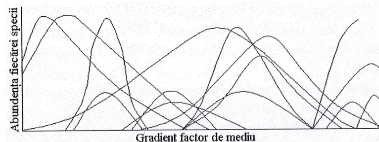
Figura 2. Tipuri ipotetice de distribuție a abundenței speciilor de-a lungul unui gradient de mediu care se modifică gradual cu o rată uniformă (adaptată după Kent, 1998).
