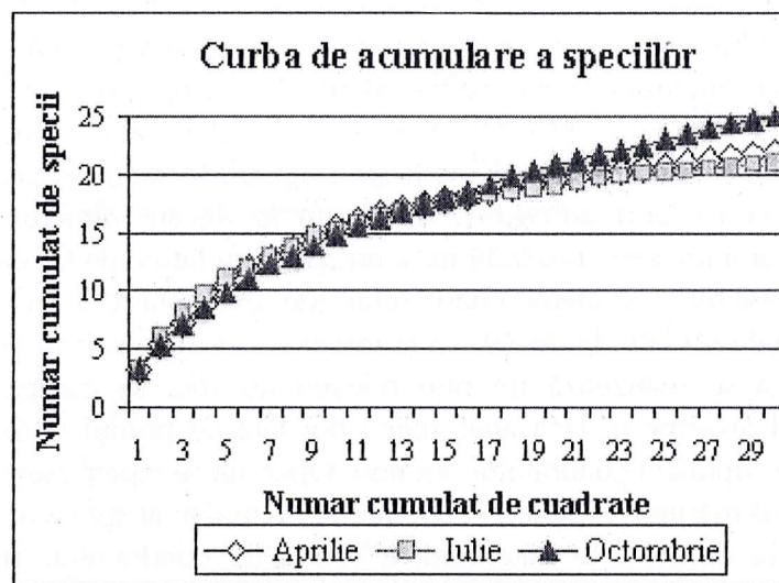
Figura 12. Curba de acumulare a speciilor pe măsură ce crește numărul de quadrate, la trei momente diferite de timp (aprilie, iulie, octombrie) (Țopa, 2003).
