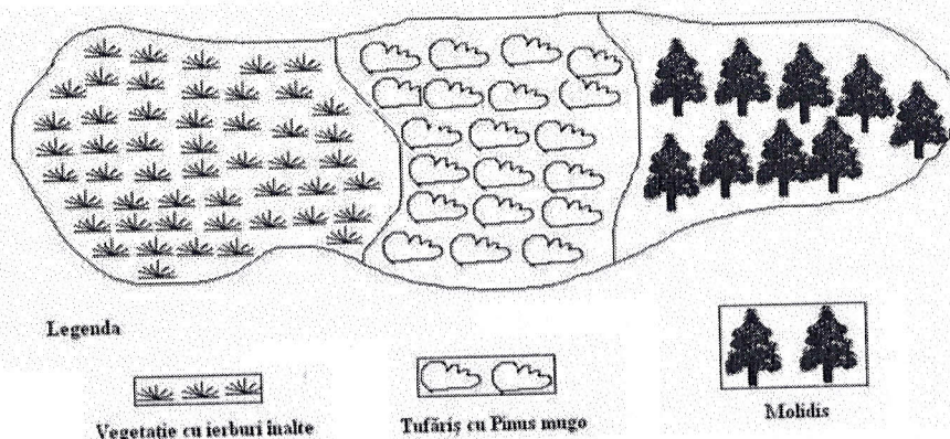
Figura 14. Harta de vegetație a unei zone în care sunt prezente trei tipuri de vegetație diferite.
