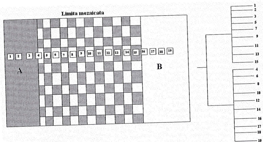
Figura 4. Gruparea cuadratelor situate pe un transect care străbate limita mozaică și porțiuni relativ reduse din comunitățile (A,B) adiacente, separate între ele prin limită mozaică.
