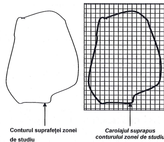
Figura 13. Metoda caroiajului, stabilirea poziționării quadratelor.
