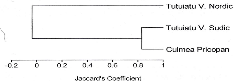
Figura 5. Cluster-ul obținut prin prelucrarea matricei transpuse, prezentă în tabelul 2, folosind programul MVSP.
