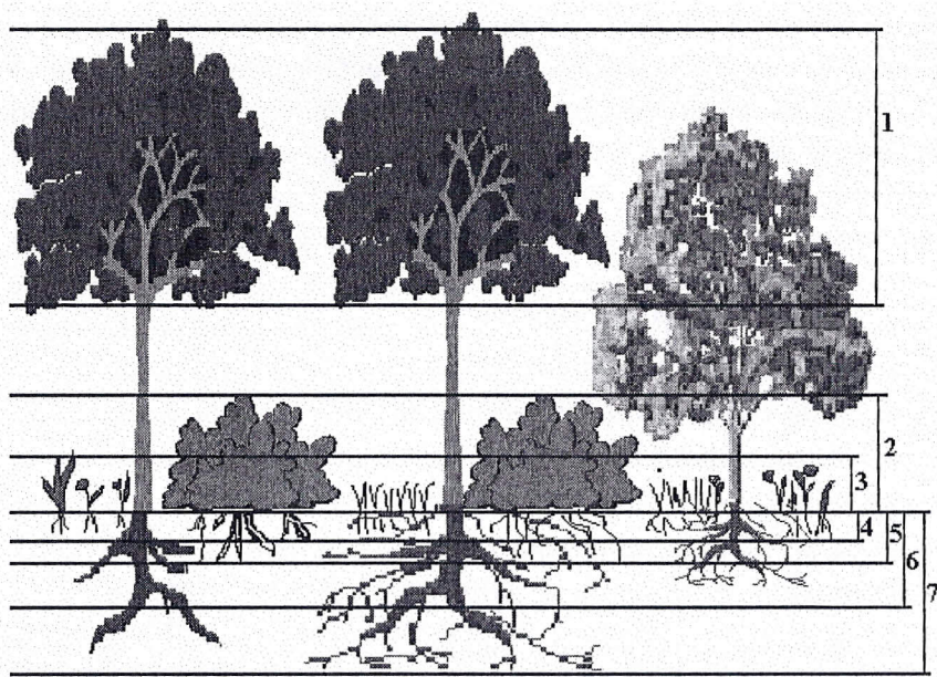
1. Stratul arborilor; 2. Stratul arbuștilor; 3. Stratul ierburilor; 4. Stratul de rizomi și bulbi; 5. Stratul rădăcinilor superficiale de arbuști și arbori; 6. Stratul rădăcinilor mijlocii de arbori; 7. Stratul rădăcinilor profunde de arbori.
