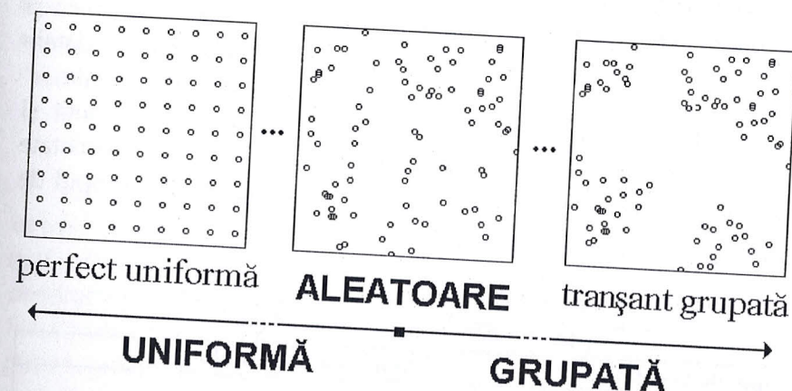
Figura 10. Modelele fundamentale de distribuție a vegetației în teren (Dragomirescu, 1993 – reprodusă cu permisiunea autorului).
