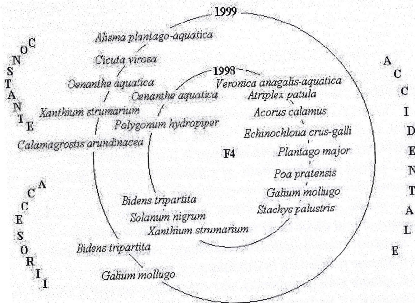
Figura 8. Diagrama speciilor constante, accesorii și accidentale.
