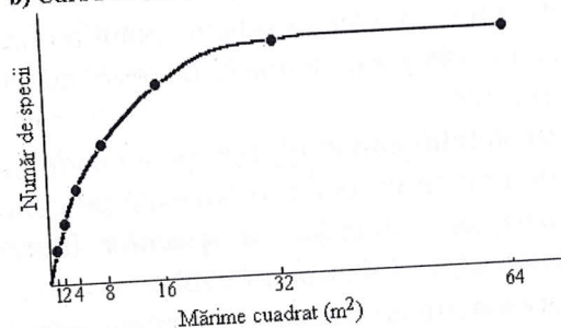
Figura 11. Stabilirea mărimii cuadratului: dublarea progresivă a suprafeței (a) și curba de acumulare a speciilor (b).
