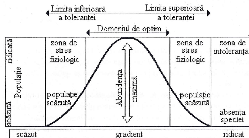
Figura 1. Curba distribuției normale (Gauss) a unei specii de plante sub acțiunea unui factor de mediu (adaptată după Kent & al, 1998). Există un domeniu optim al factorului de mediu în care populația speciei de plante are cea mai mare abundență, spre limitele domeniului de toleranță plantele găsindu-se într-o zonă de stres fiziologic, populația fiind mult redusă și lipsind în zonele în care factorul de mediu este la cele două extreme.
